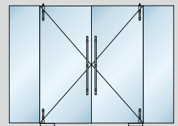
Anlagentyp 8 (2 Sets)
